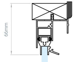
Interlock
